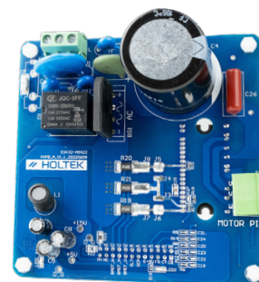
HVPB AC 90 ~ 264 V / 2.5 A
